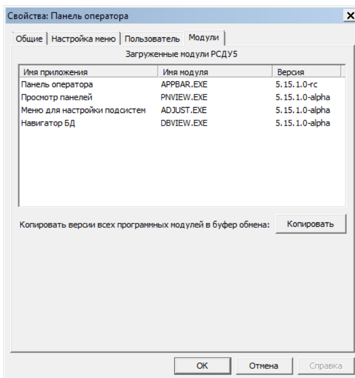
Рисунок 12 – Окно свойств на вкладке «Модули»
