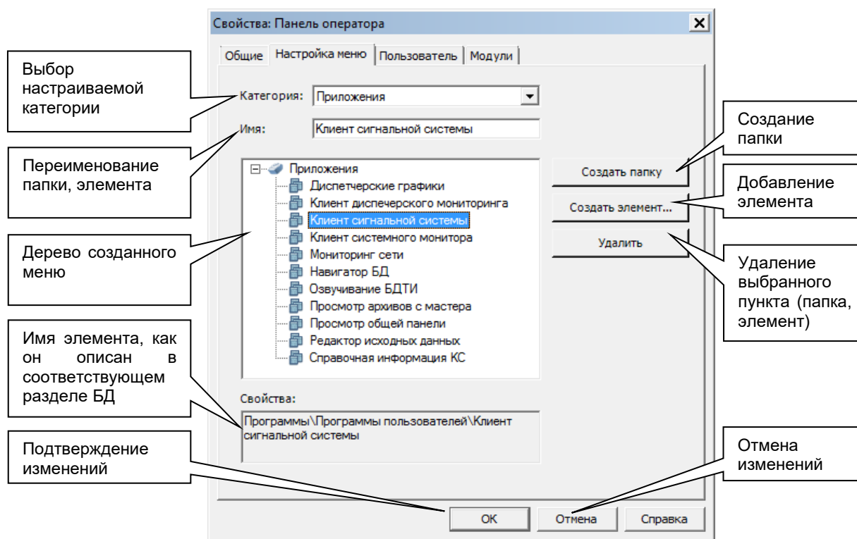
Рисунок 6 – Окно свойств на вкладке «Настройка меню»
