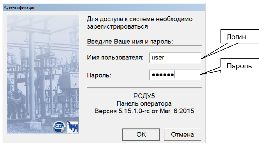
Рисунок 1 – Диалог аутентификации
